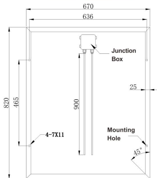
背面图
